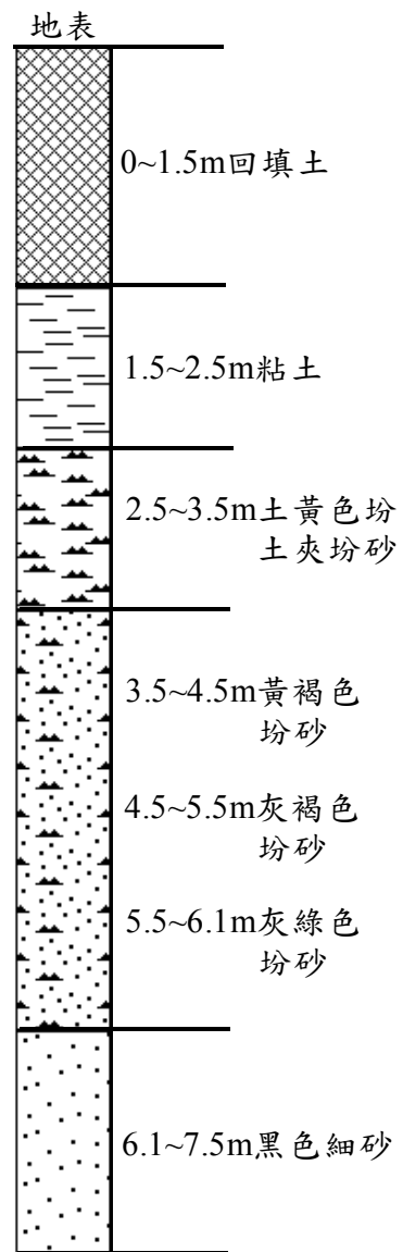
地質剖面圖
